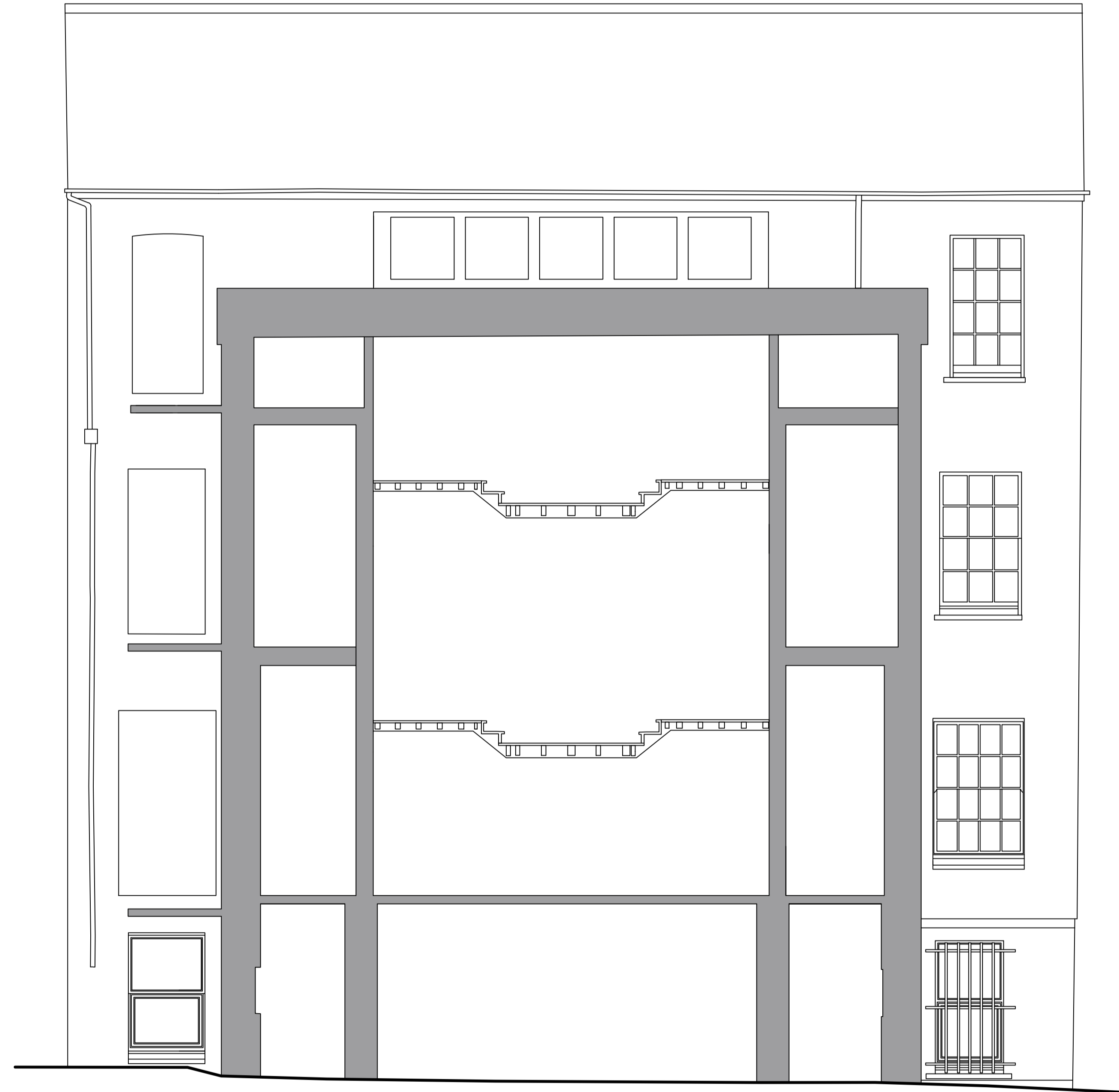
Section D - 1:50
