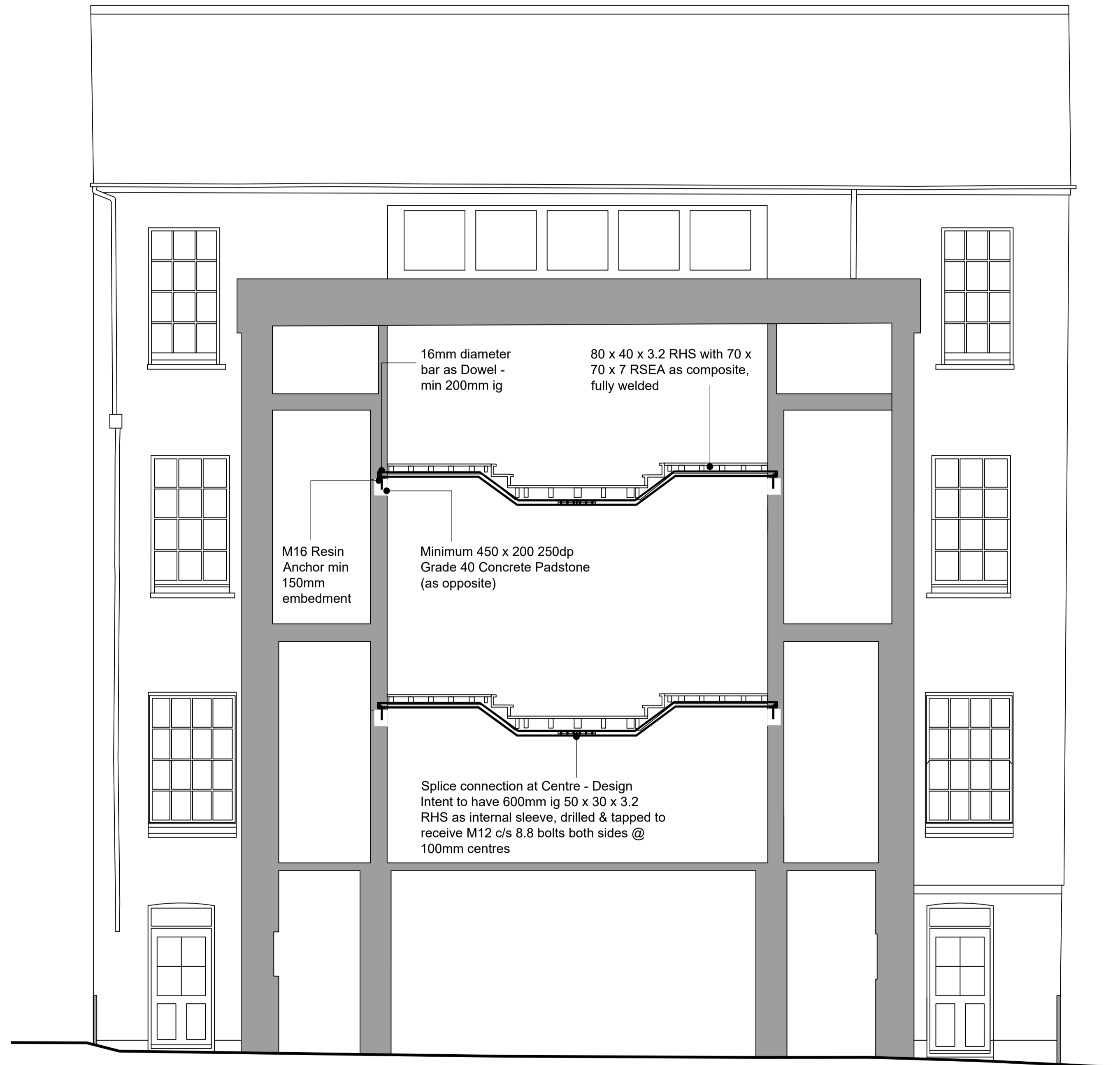
Section D - 1:50
