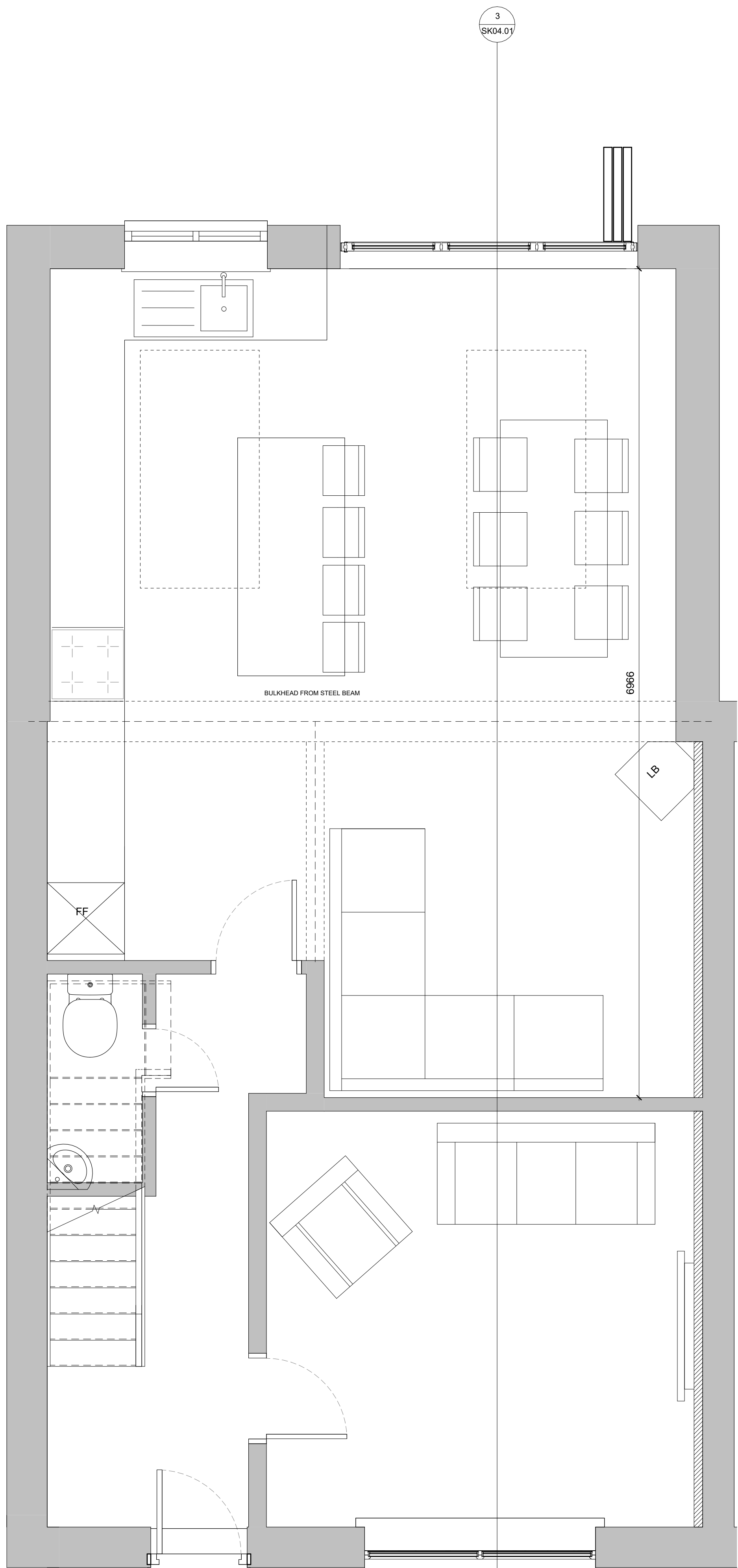
GF - PRO 1 : 25
