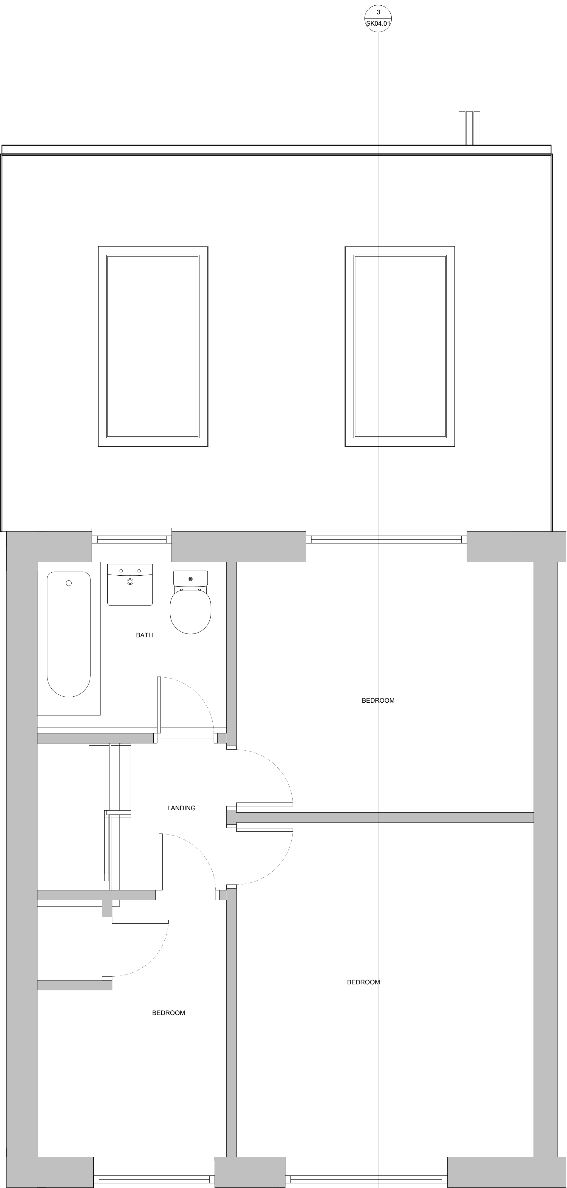
FF S04 1 : 25
