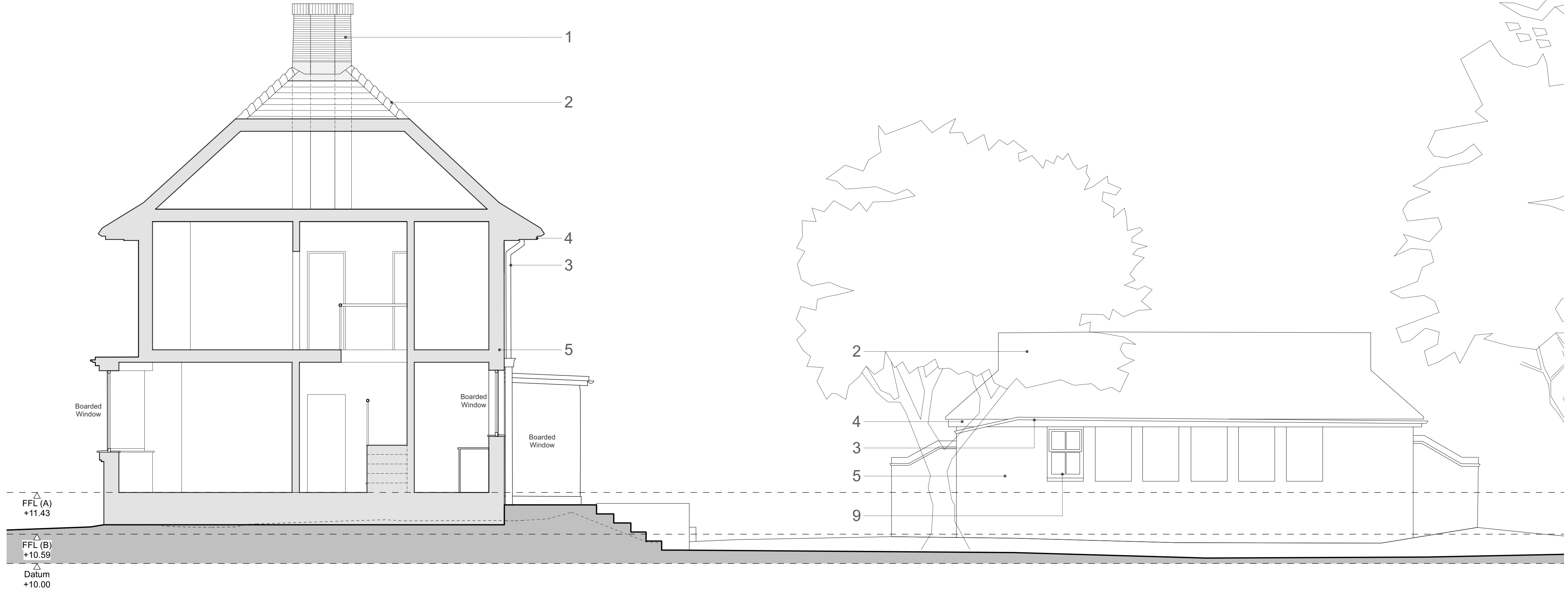
Cross Section 01 Scale: 1:50
