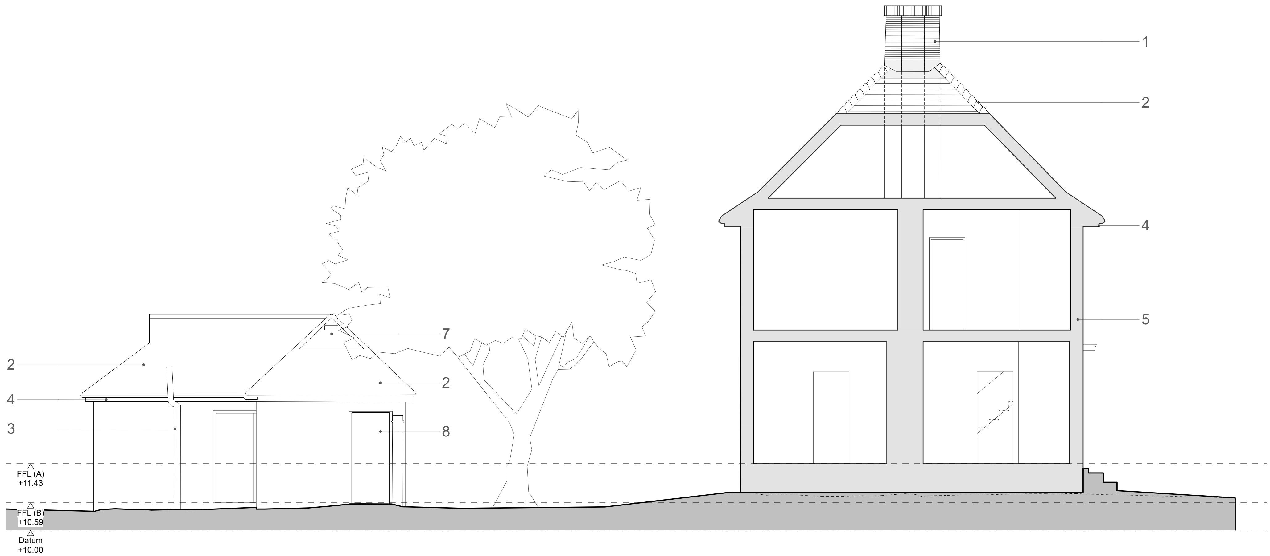
Cross Section 02 Scale: 1:50
