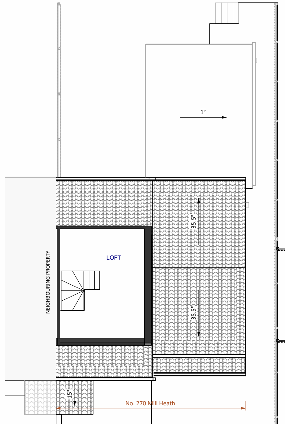
Loft Floor Plan 1 : 100
