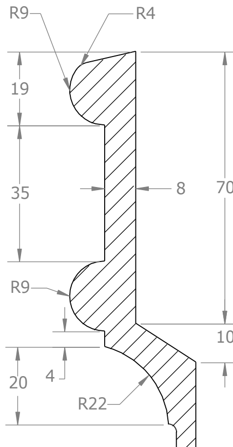
SECTION A-A SCALE 1 : 1
