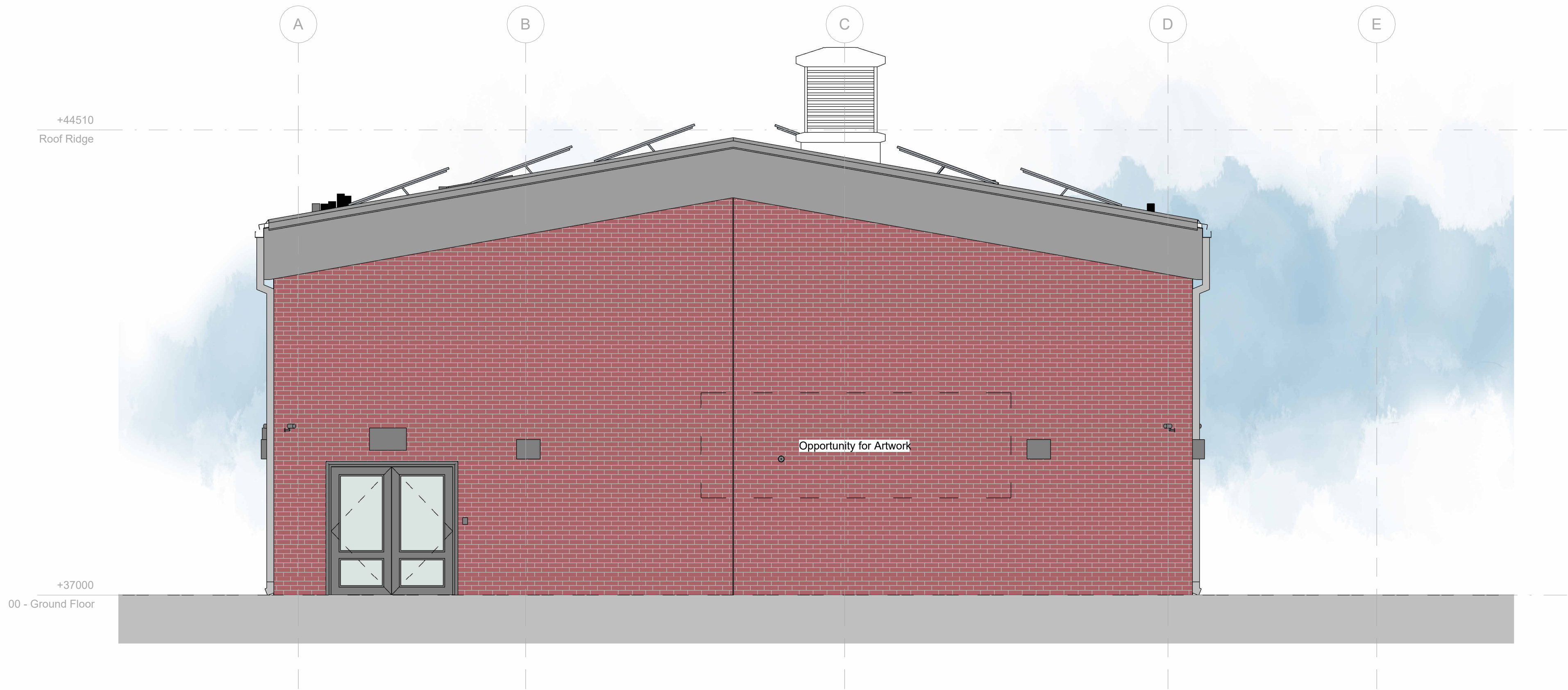
Elevation 1 Scale: 1 : 50
