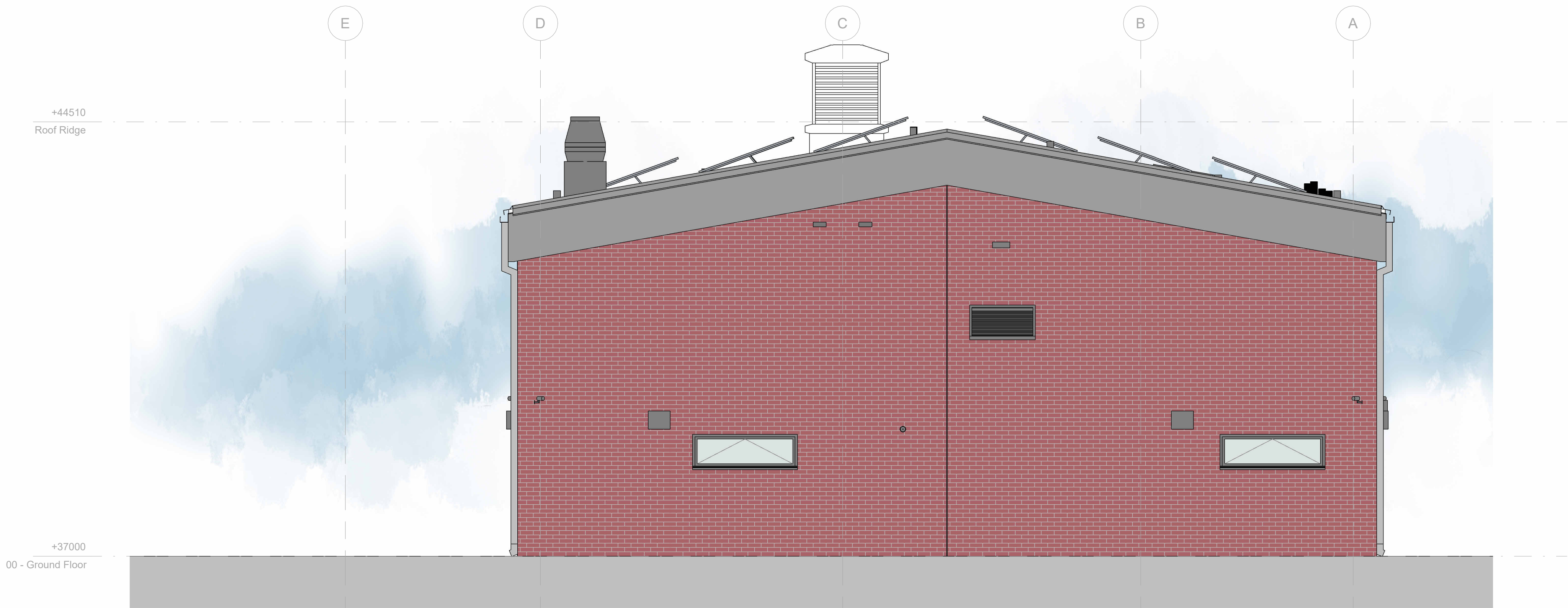
Elevation 3 Scale: 1 : 50
