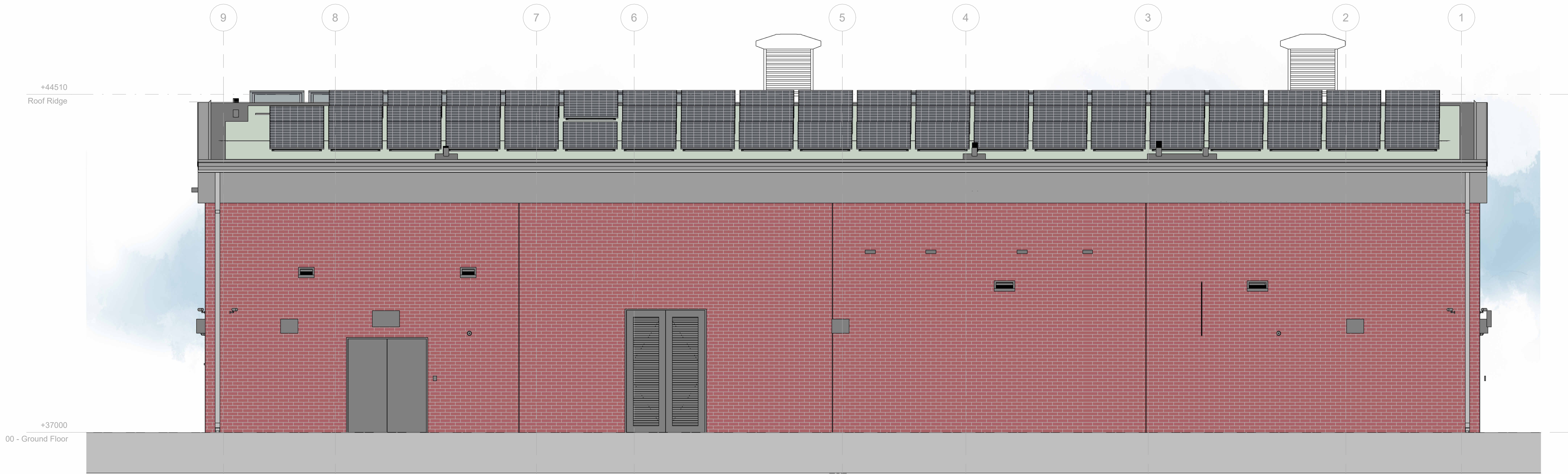
Elevation 4 Scale: 1 : 50
