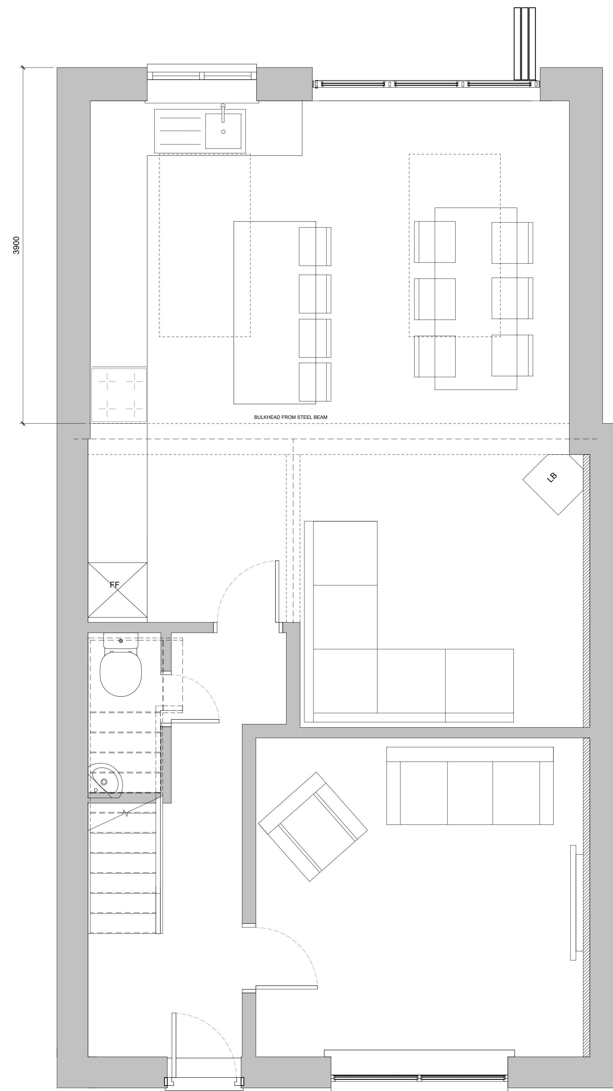
GF - PRO 1 : 25
