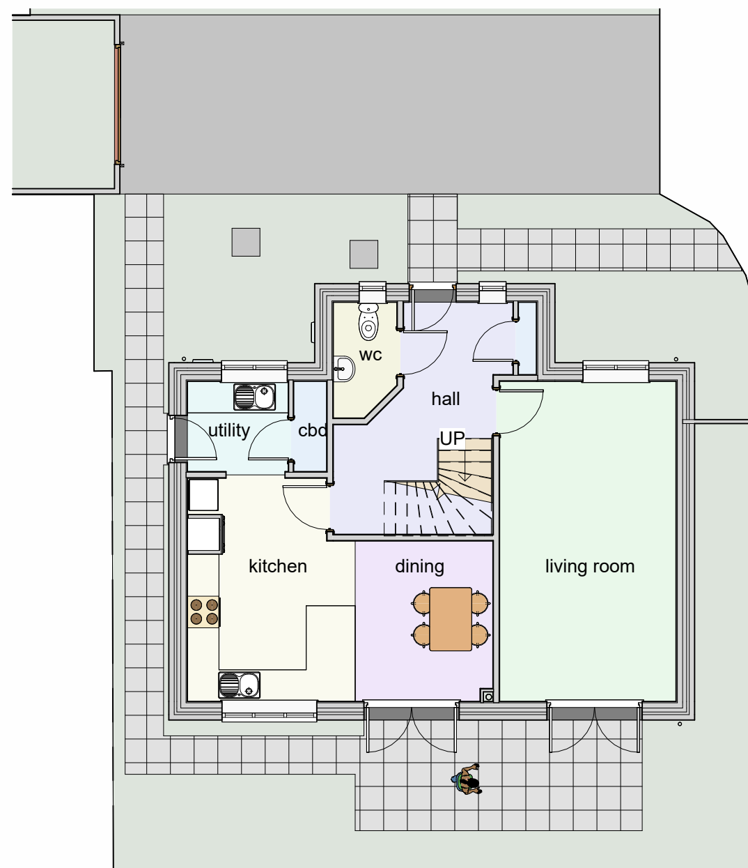
1 0_grd FFL Existing 1 : 100
