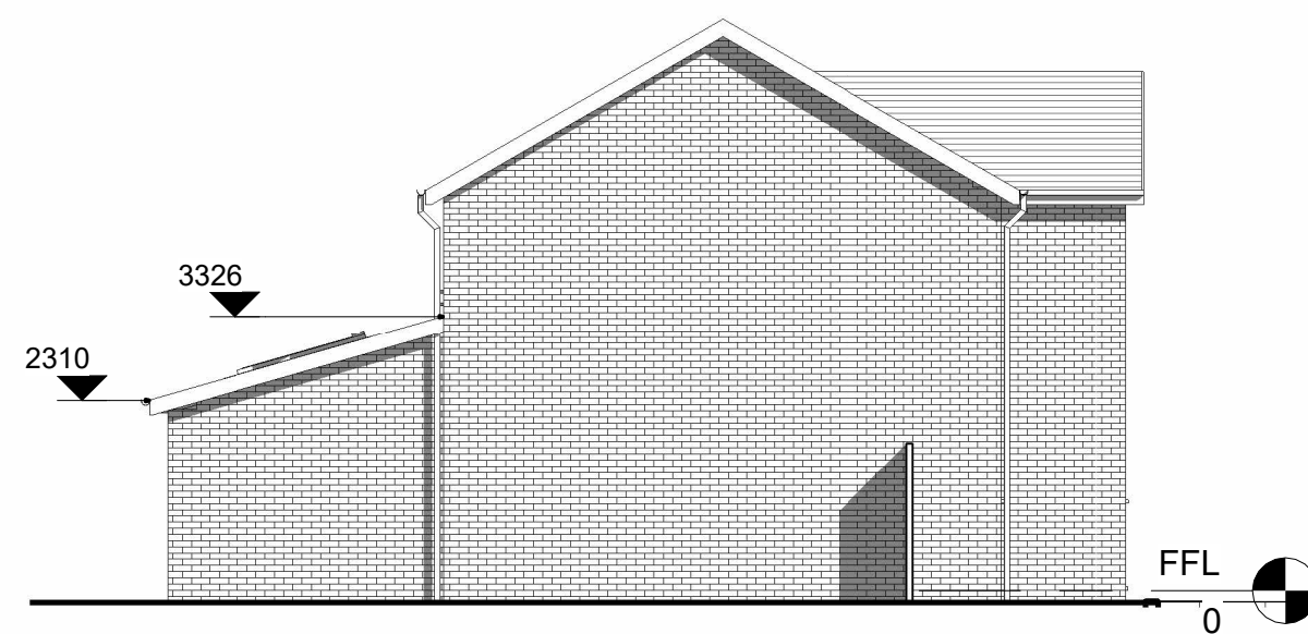
3 SIDE 1 : 100
