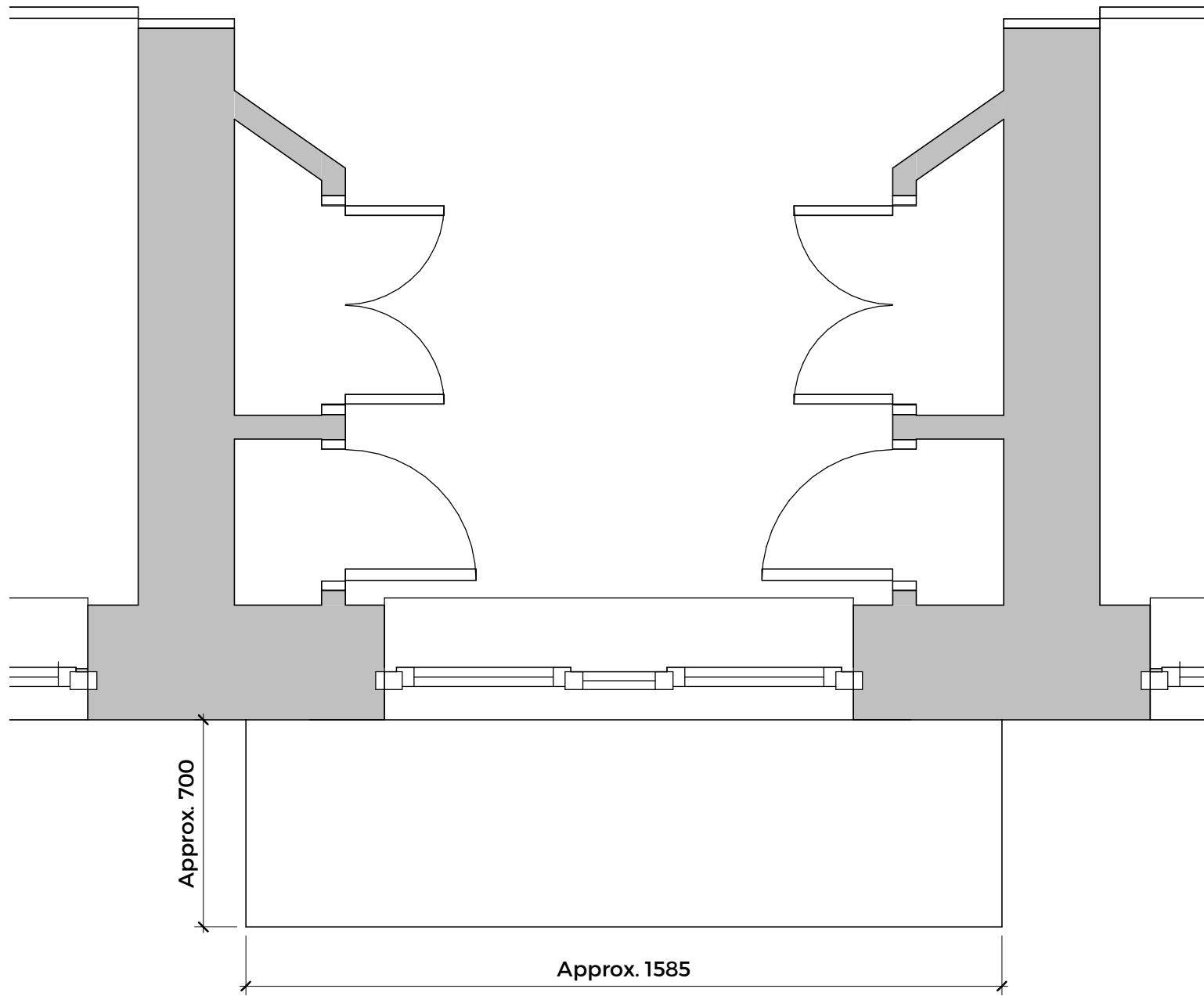
Canopy Plan 1 : 20
