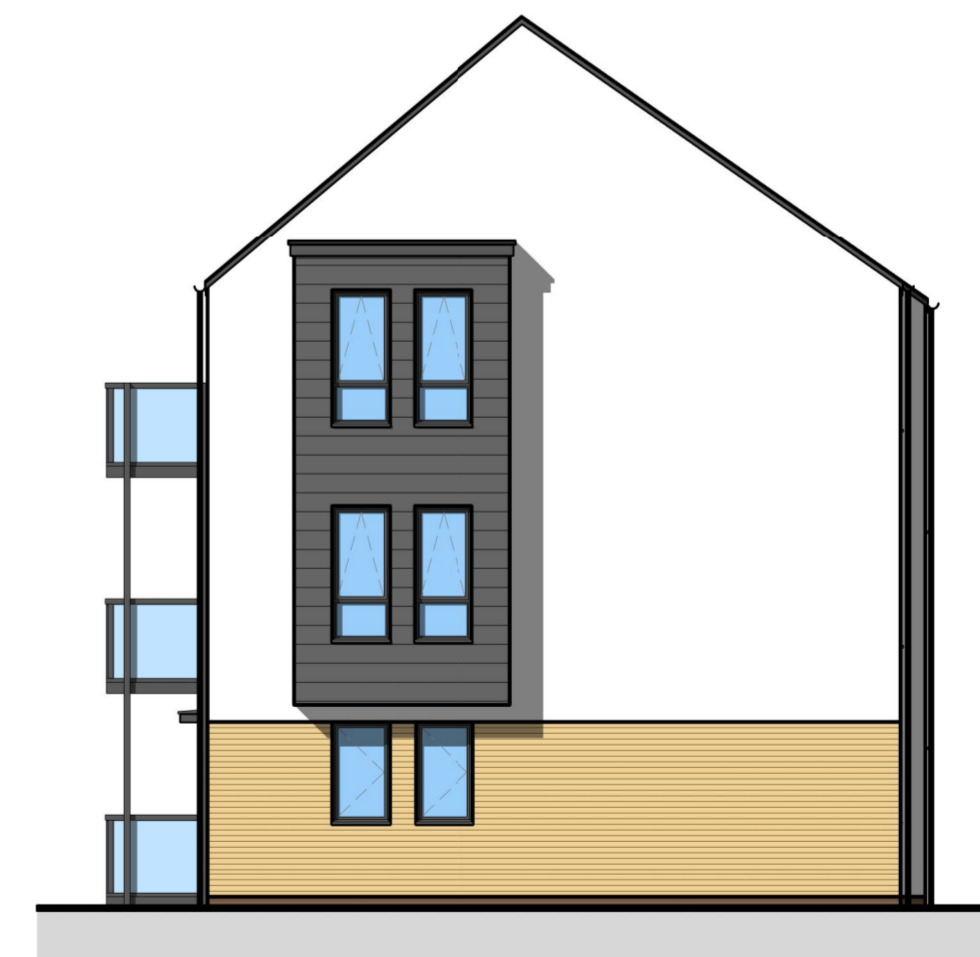
R.H.S Elevation
