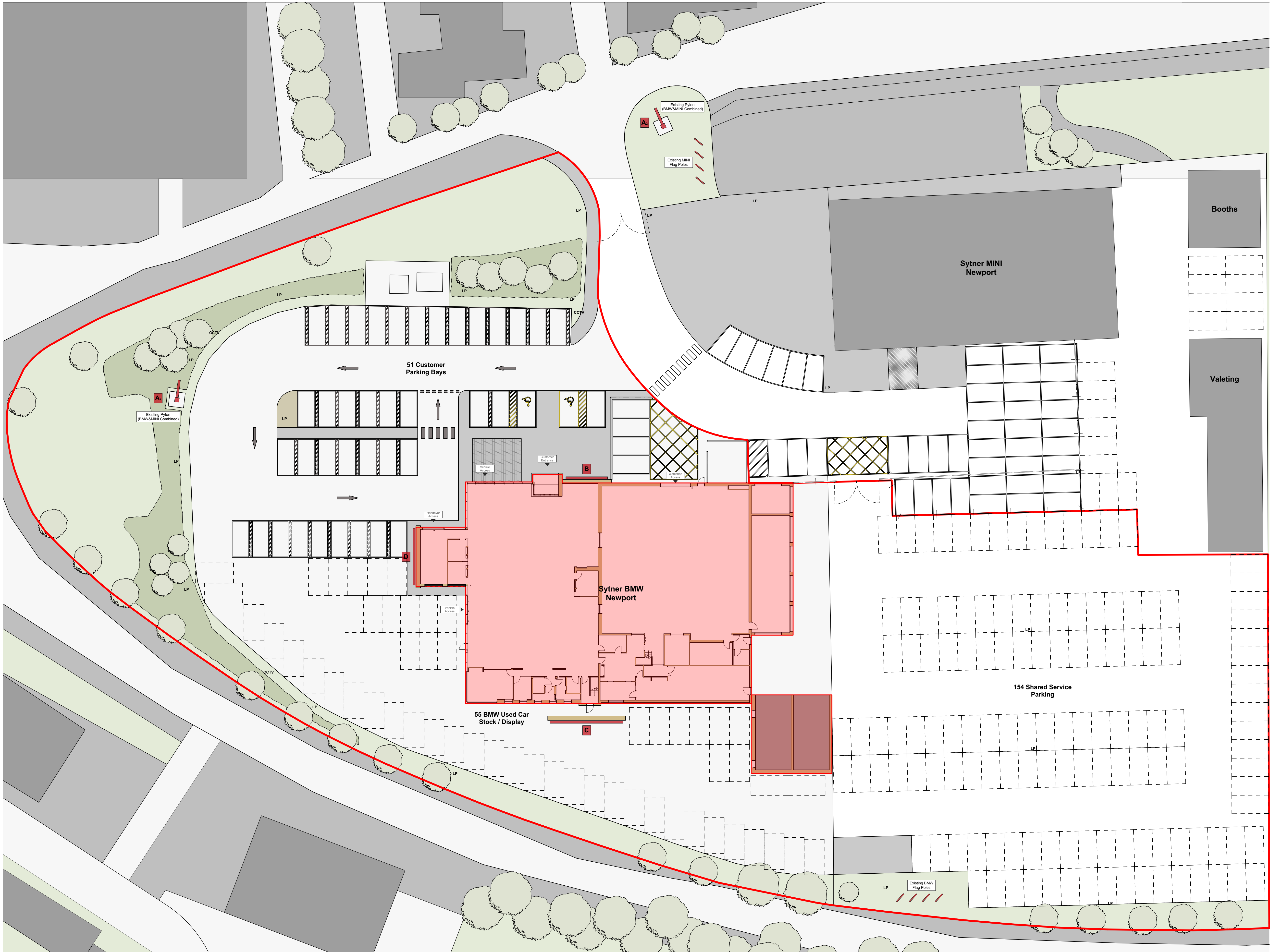
Existing Site Plan BMW 1:250
