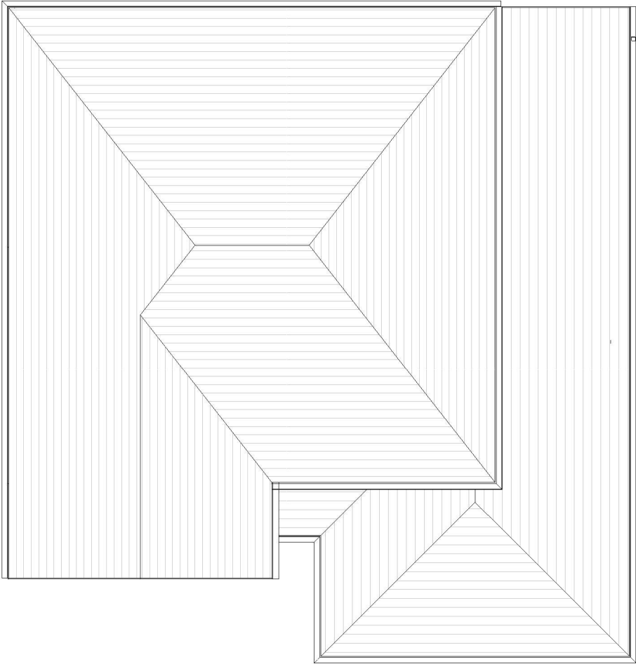
Roof plan 1 : 100
