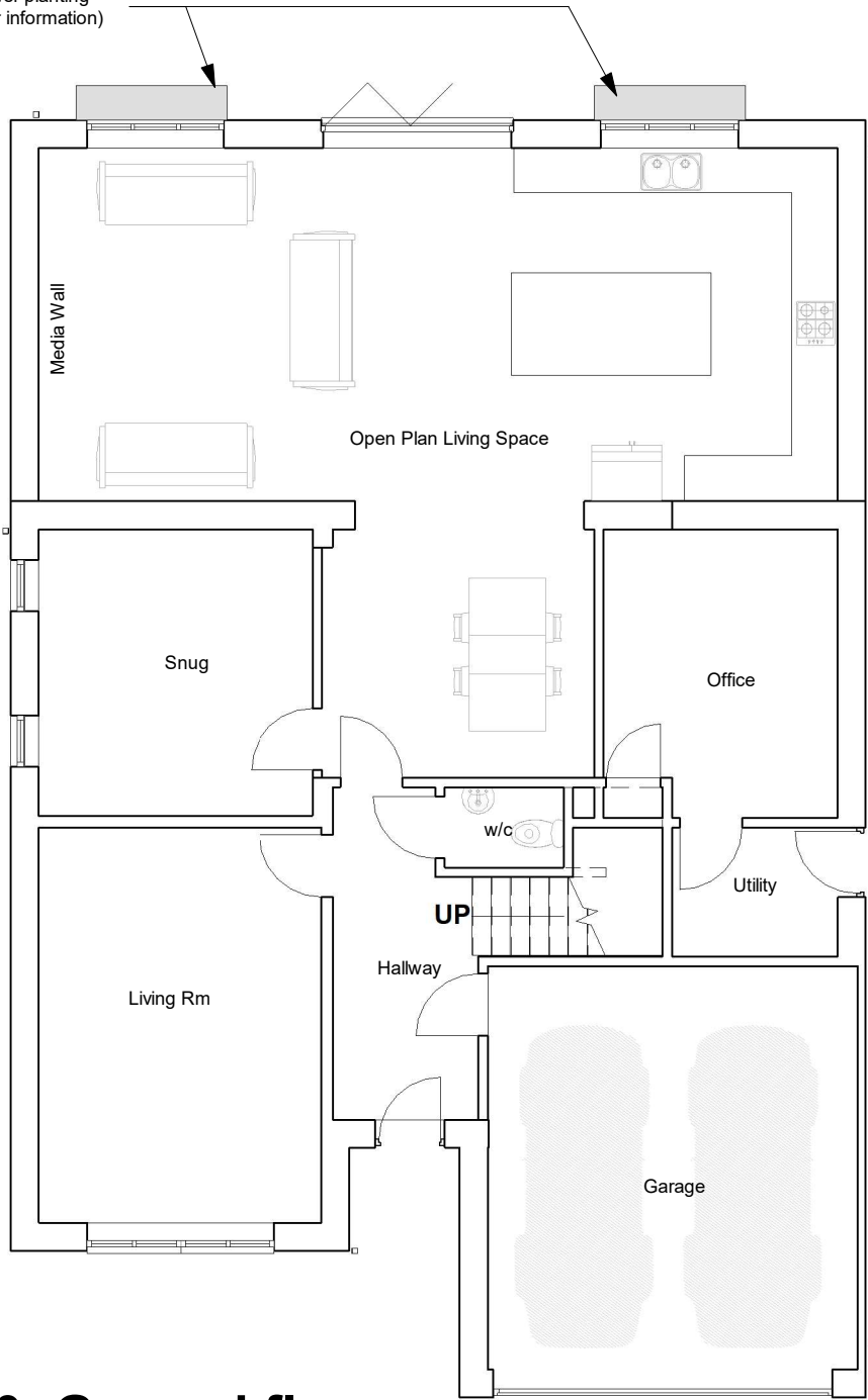
0_Ground floor 1 : 100
