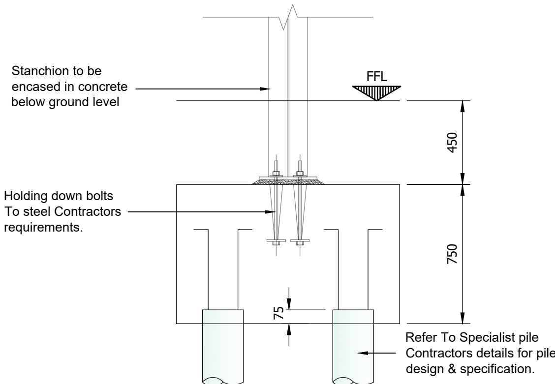
Pile Cap Type 2a Section A-A Scale 1 : 20
