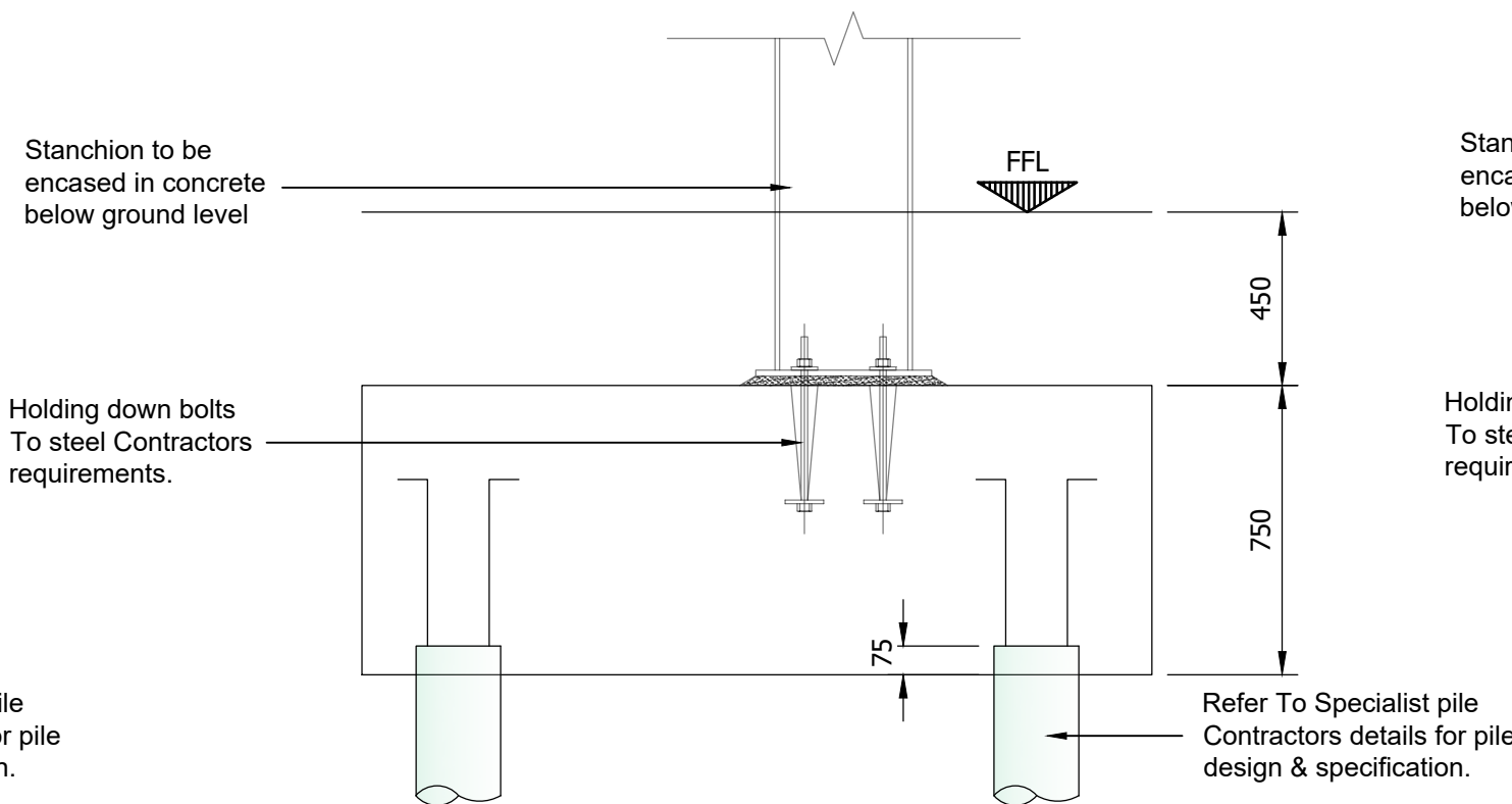
Pile Cap Type 2a Section B-B Scale 1 : 20
