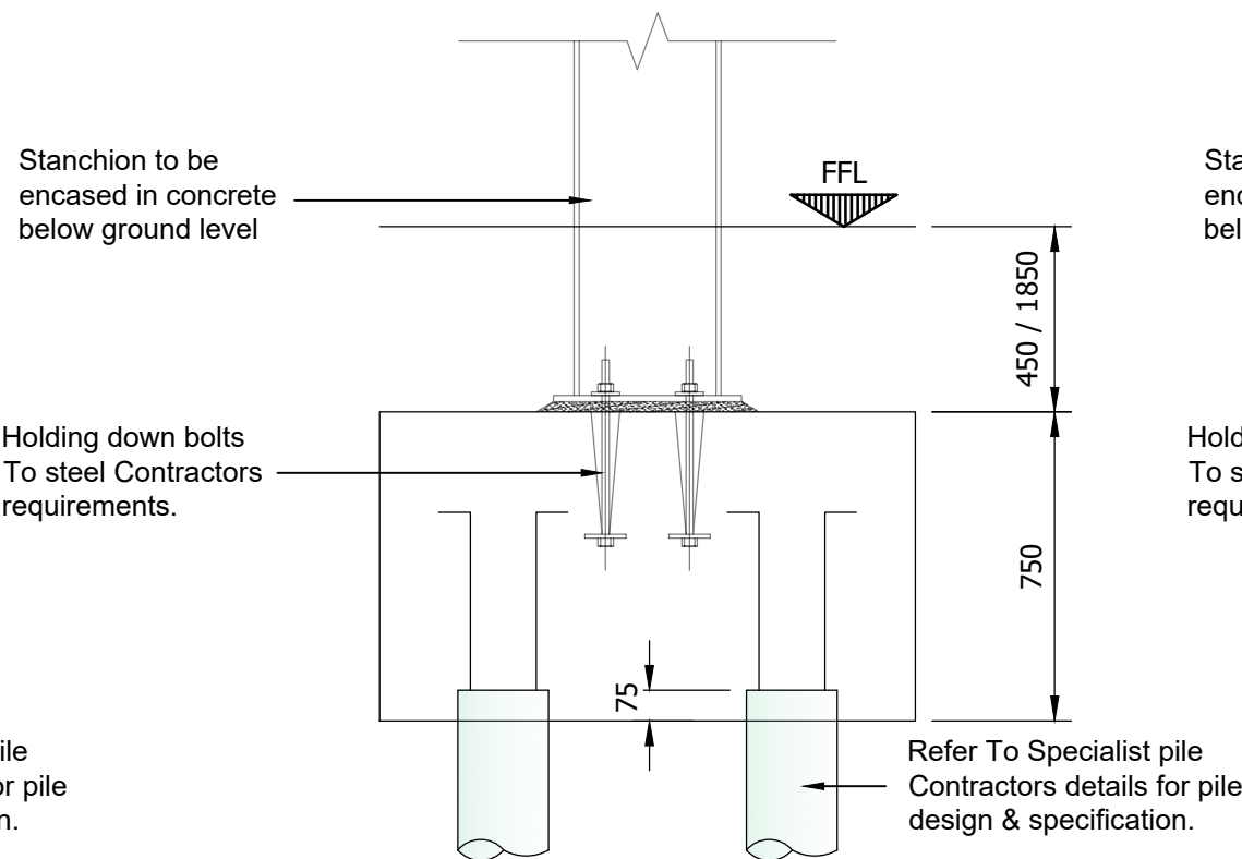
Pile Cap Type 1b Section B-B Scale 1 : 20
