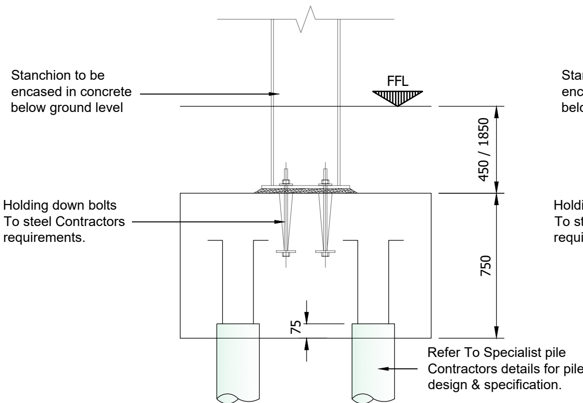
Pile Cap Type 1a Section B-B Scale 1 : 20
