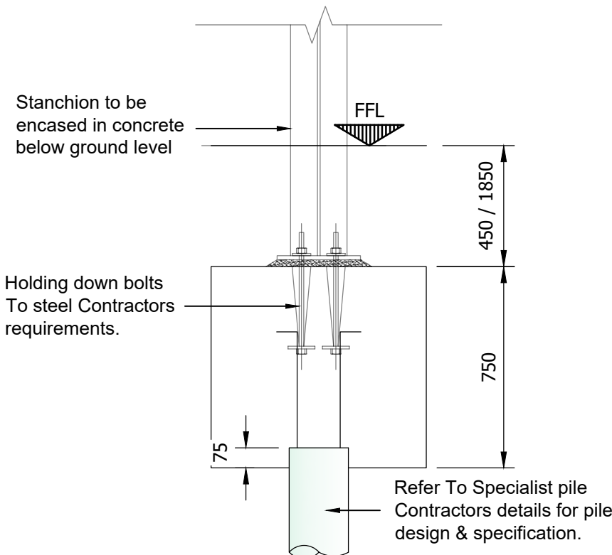
Pile Cap Type 1b Section A-A Scale 1 : 20
