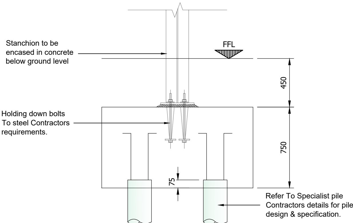
Pile Cap Type 2b Section A-A Scale 1 : 20
