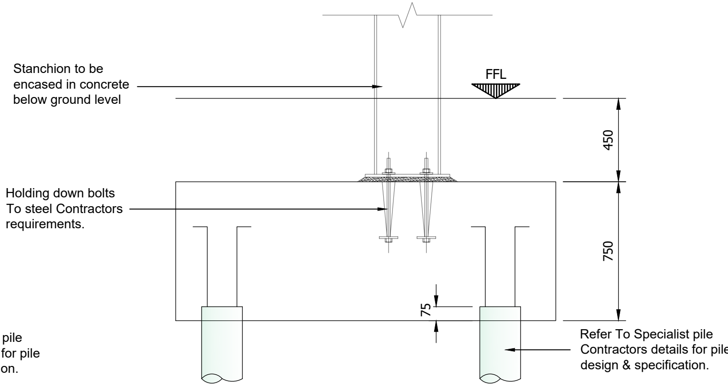
Pile Cap Type 2b Section B-B Scale 1 : 20
