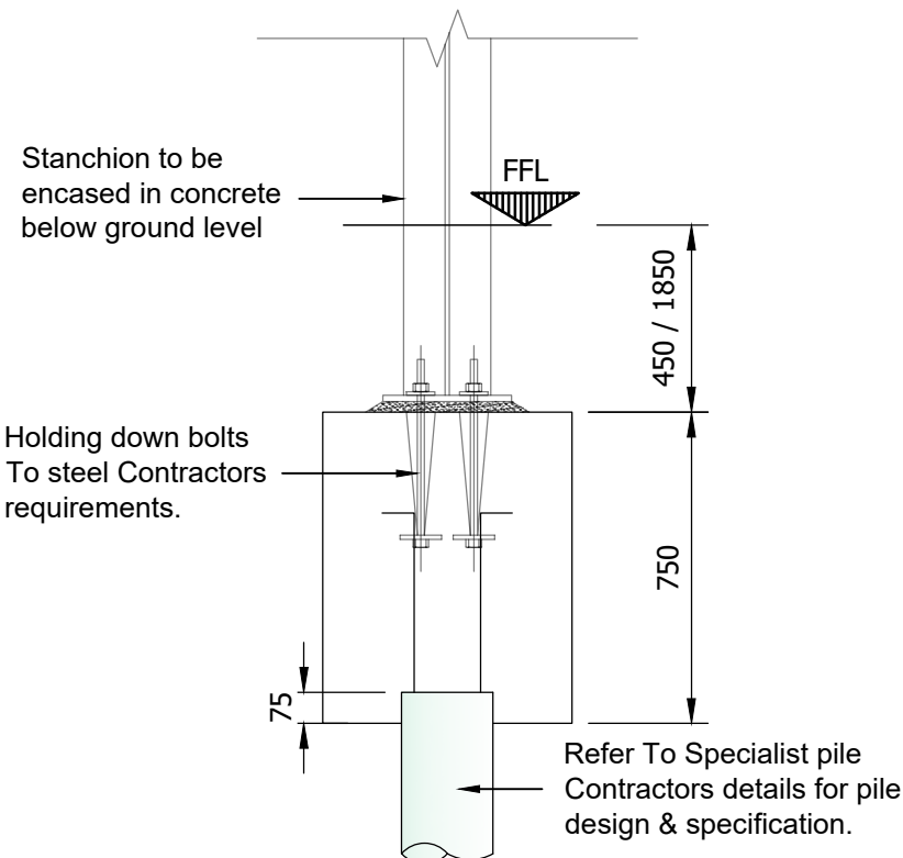
Pile Cap Type 1a Section A-A Scale 1 : 20
