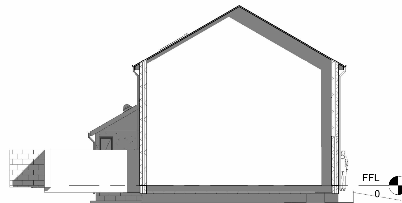
6 SIDE 1 : 100
