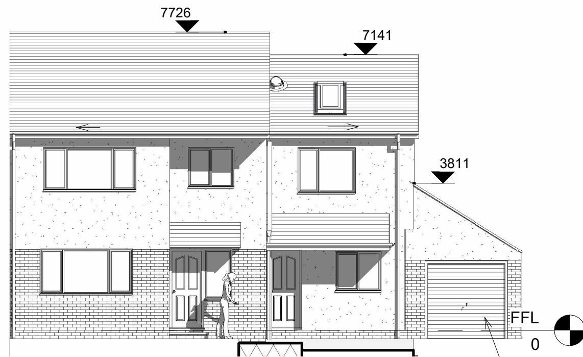
3 FRONT 1 : 100
