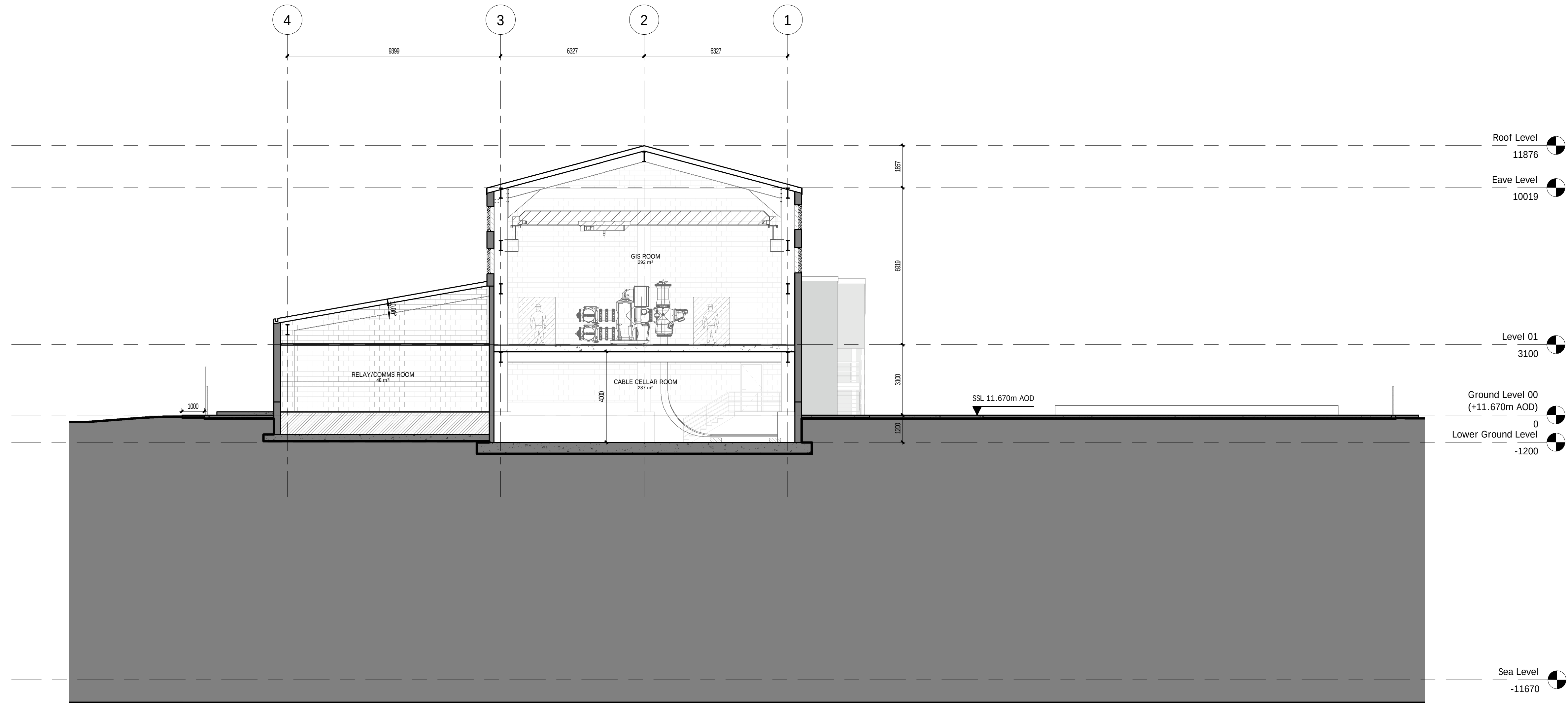
2 Section 2 1 : 100
