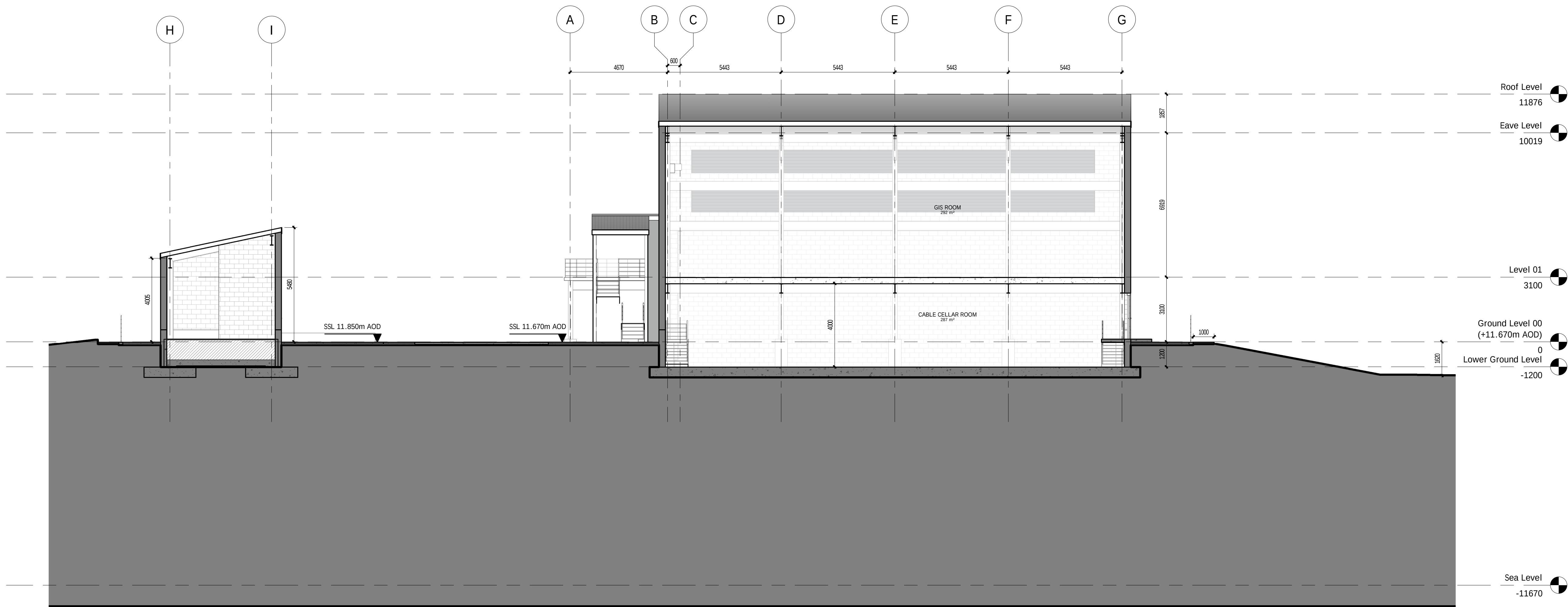
3 Section 3 1 : 100
