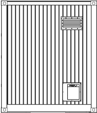
Elevation 1 1:50
