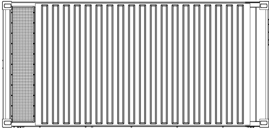
Elevation 2 1:50
