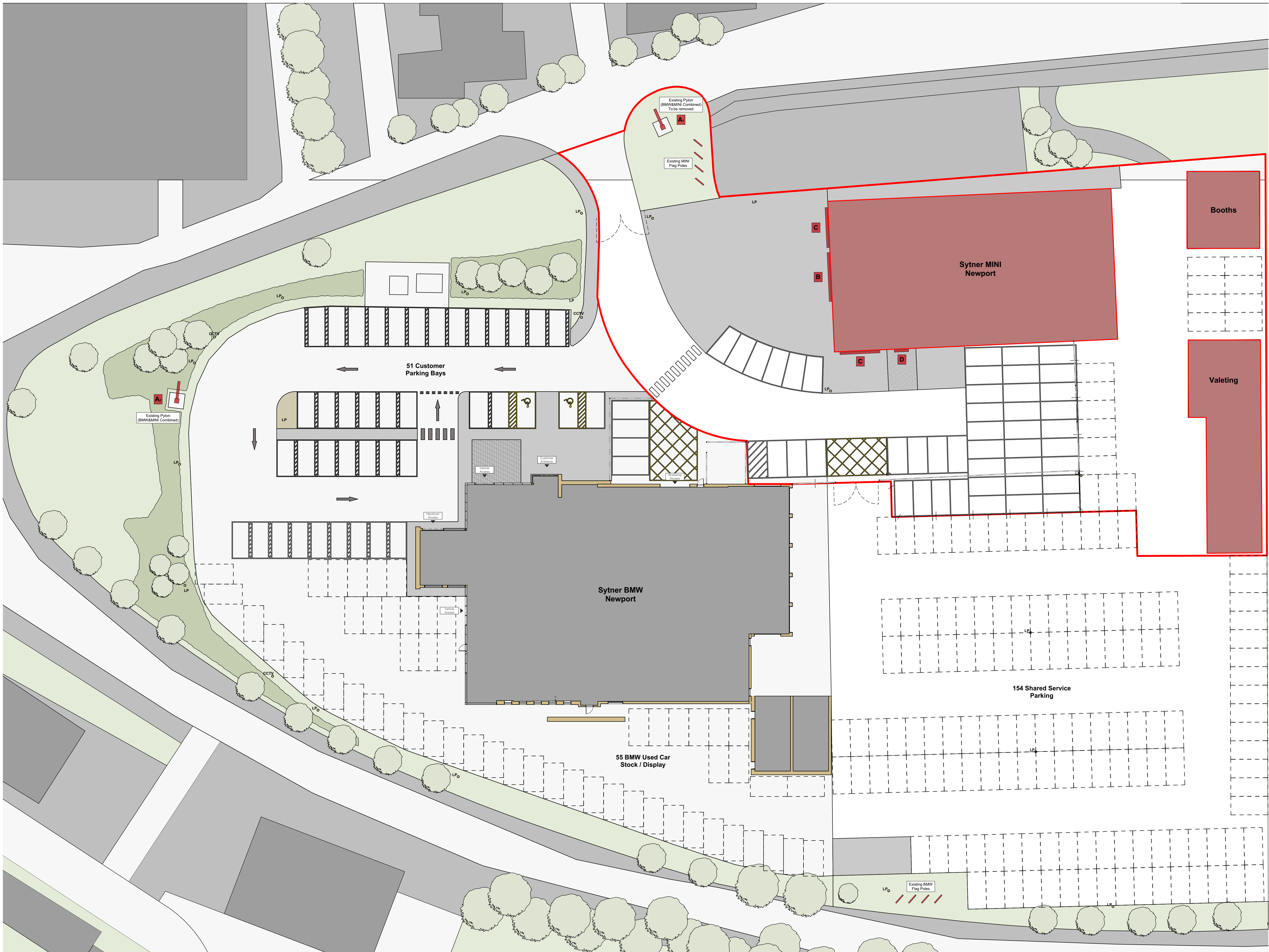
Existing Site Plan MINI 1:250
