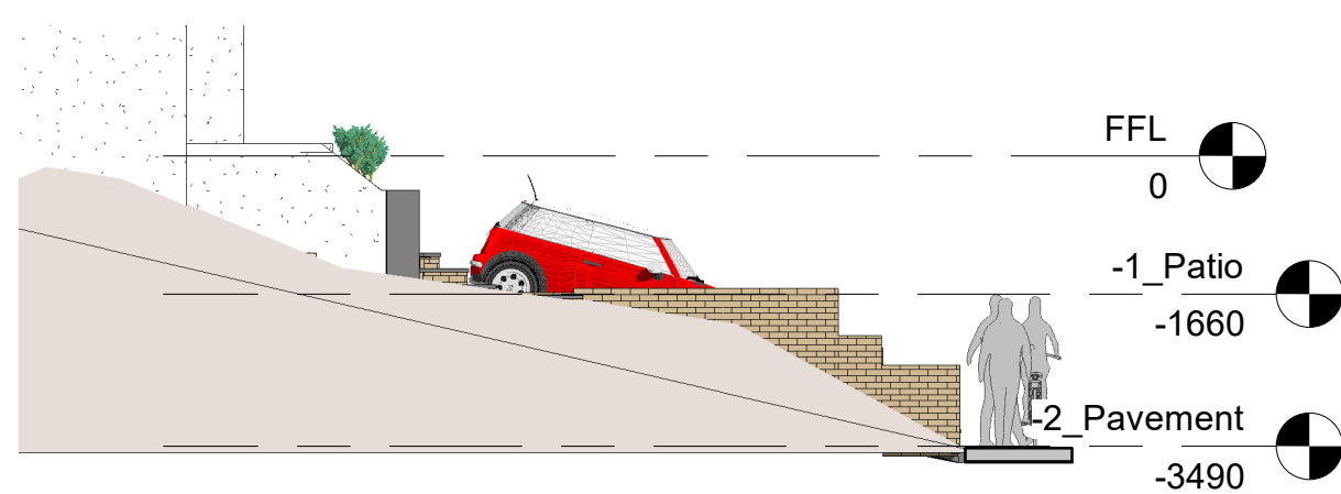
4 SIDE 1 : 100
