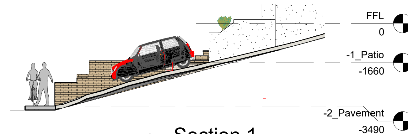
6 Section 1 1 : 100
