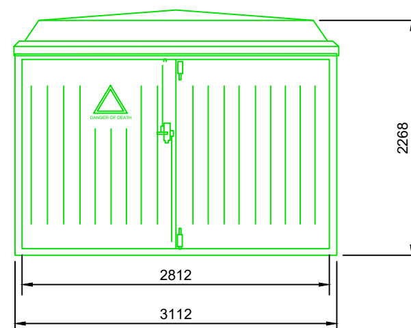
Right Elevation
