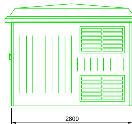
Right Elevation
